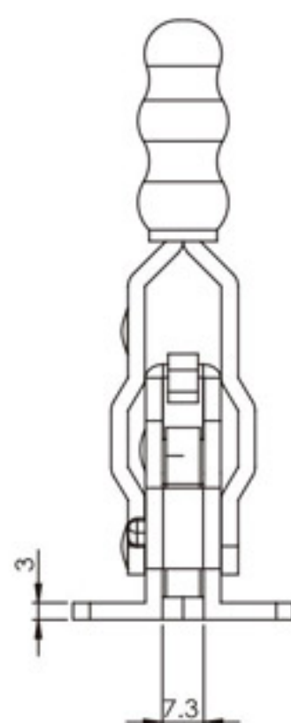
不鏽鋼,95公斤夾特力 Stainless Steel,95kg Holding capacity
