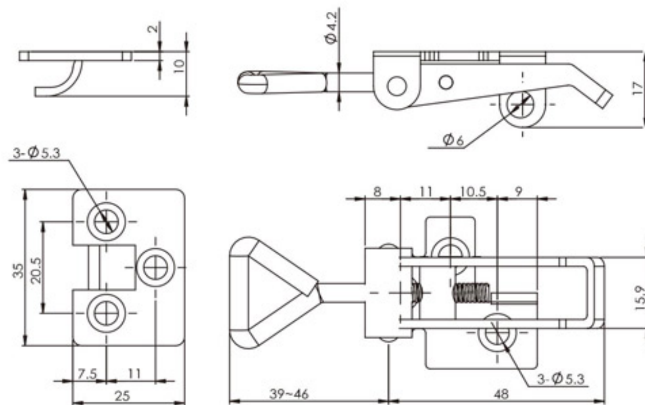
不鏽鋼 304, 震動處理 Stainless steel 304, Vibration grind
