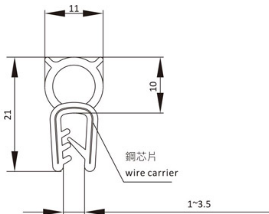
黑色發泡EPDM密封膠條 Sponge-rubber,Black EPDM gasket
