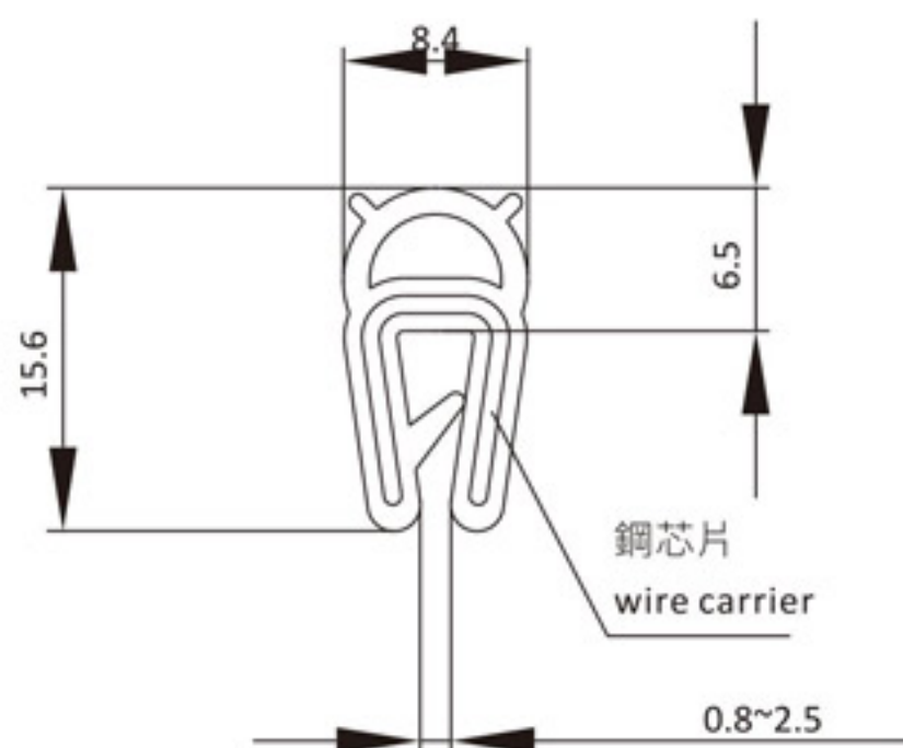
黑色發泡EPDM密封膠條 Sponge-rubber,Black EPDM gasket
