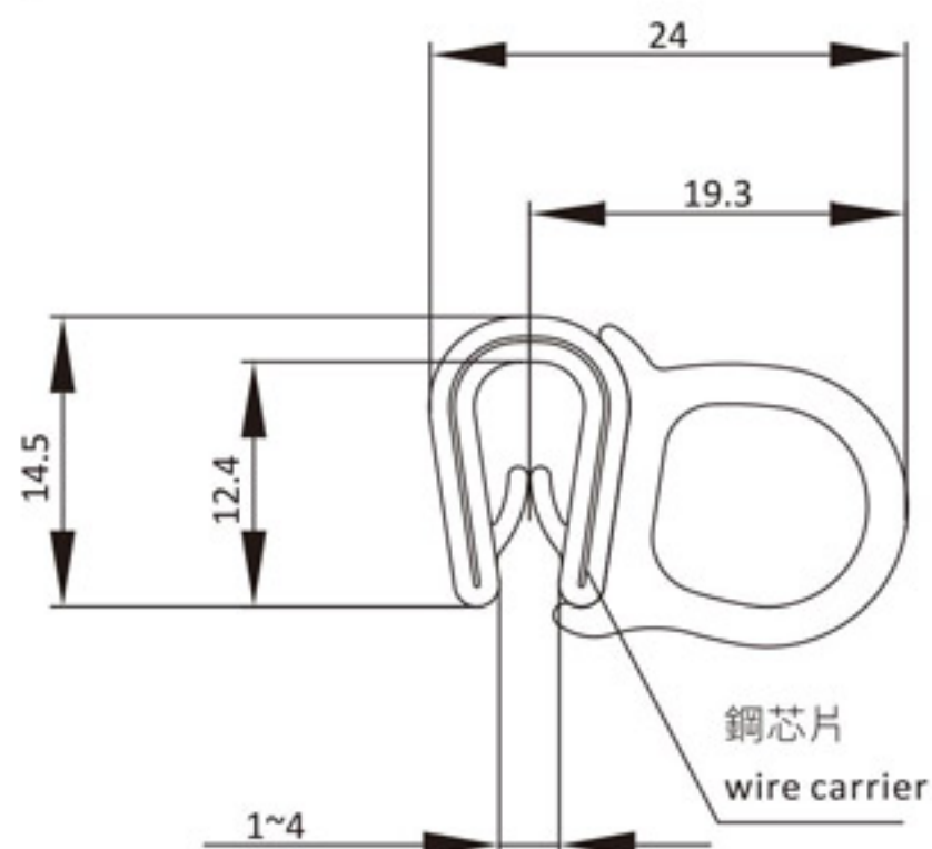
黑色發泡EPDM密封膠條 Sponge-rubber,Black EPDM gasket
