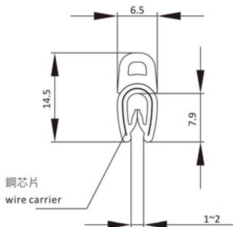
黑色發泡EPDM密封膠條 Sponge-rubber,Black EPDM gasket
