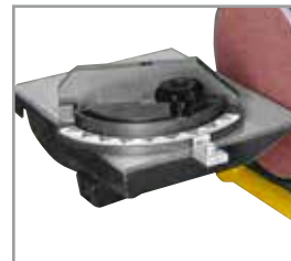
Workbench with goniometer and 150 mm disc for sanding curved workpieces or angular ends. Mesa de trabajo con goniómetro y 150 mm de disco abrasivo para pulir piezas curvadas o para trabajar los extremos angulares.
