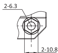
A部剖視圖
