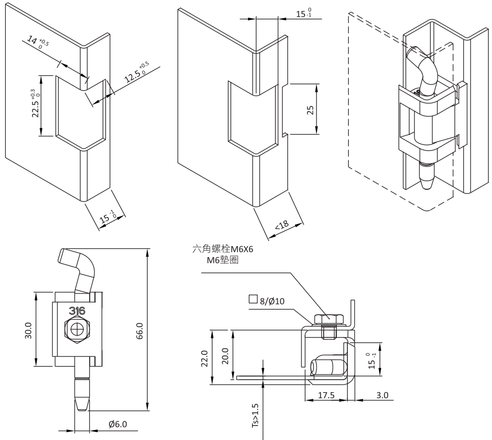
180°不鏽鋼SUS 316鉸鏈,不鏽鋼銷軸 180° hinge SUS 316, pin SUS 304
