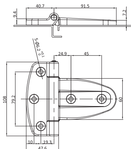
黑色PA+GF鉸鏈, 不鏽鋼銷軸 Hinge Polyimide GF 30% black, M.S. zinc plated pin
