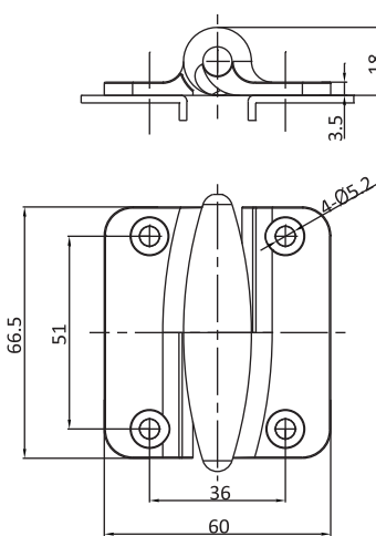
R型 (右裝) Version R(Right) B-2115-76604-R
