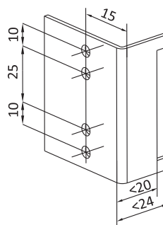
開孔尺寸 Panel cutout
