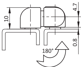
右裝型 Right
