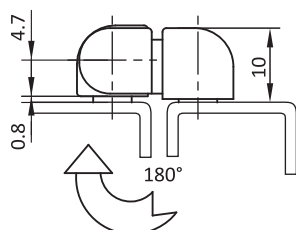
左裝型 Left
