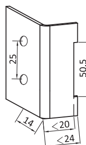
開孔尺寸 Panel cutout
