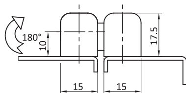
左裝型 Left
